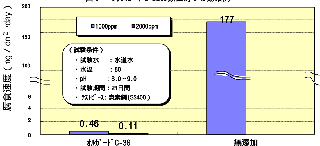
図. オルガ-ドC-3Sの鉄に対する効果例
